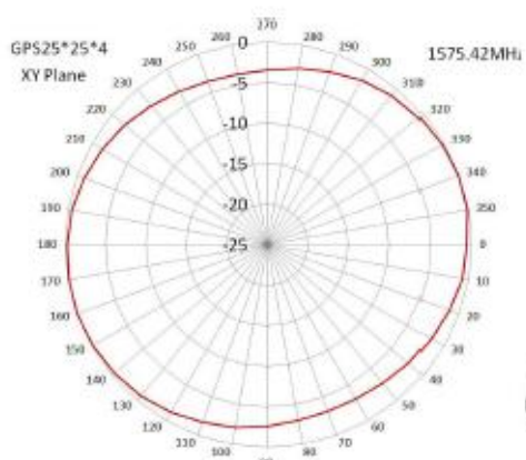
GPS Antenna
