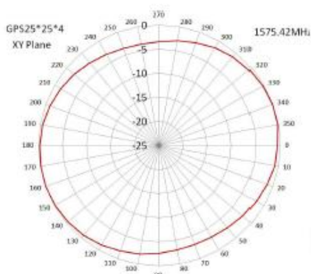
GPS Antenna
