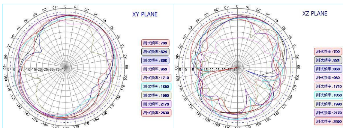
LTE Antenna
